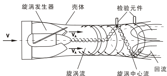
工作原理图
