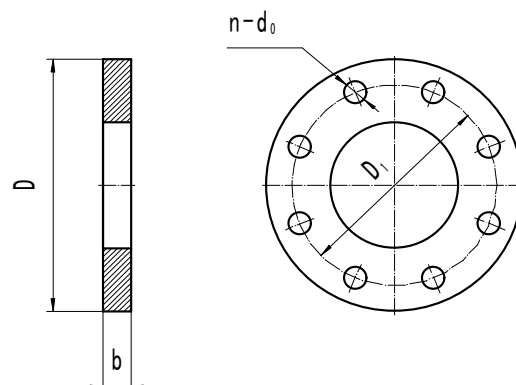
连接法兰
